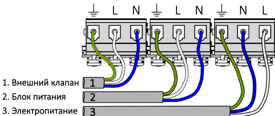
Рис. 4 Клеммная колодка
