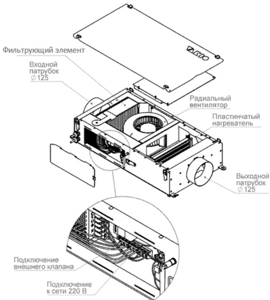
Рис. 1 Общий вид и внутреннее устройство приточной установки
