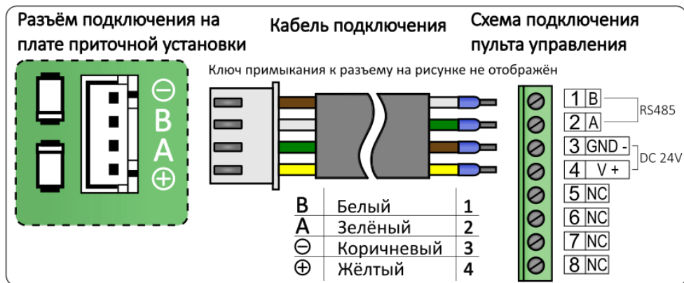
Рис. 5 Схема подключения пульта управления*
