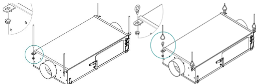
Рис. 3 Варианты монтажа вентиляционной установки
